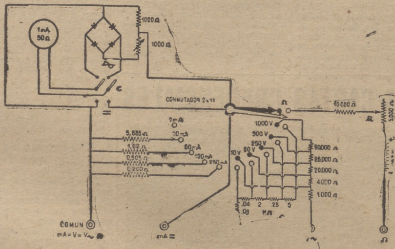
Fig. 164.—Esquema del analizador de circuitos, tester.
