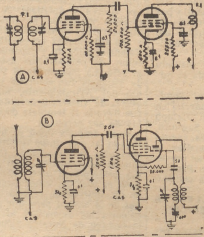
Fig. 160.—Pasos amplificadores de R. F. acoplados a resistencias.
