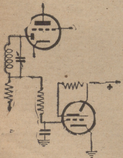
Fig. 138.—Esquema de conexión del "Ojo mágico"
