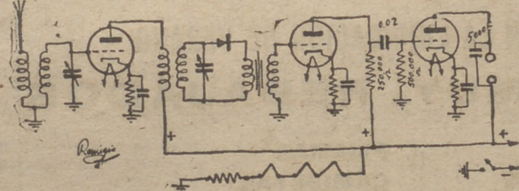
Fig. 106.—Esquema del receptor que presenta Remigio
