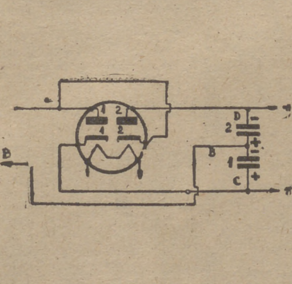
Fig. 104.—Circuito rectificador con lámpara de cátodo frío
