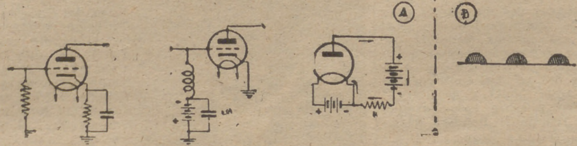
Fig. 88: Polarización de rejilla automática por cátodo.—Fig. 89: Polarización de rejilla "independientes".—Fig. 90: Sentido de la corriente electrónica rectificada
