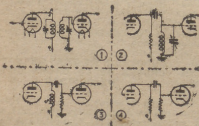
Fig. 85.—Diversos acoplamientos en alta frecuencia
