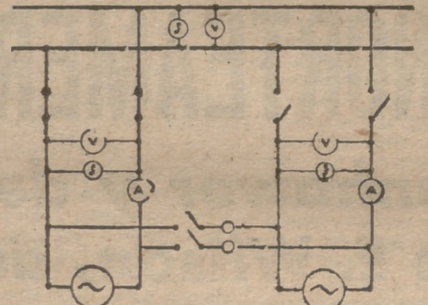
Esquema de acoplamiento en paralelo de dos alternadores monofásicos.
