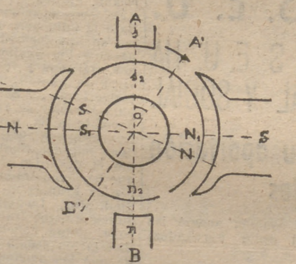
Reacción de inducido y polos de conmutación.
