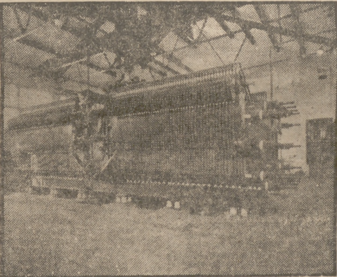
Gigantescos acumuladores instalados frente al mar recogerán la energía producida por el movimiento de las olas
