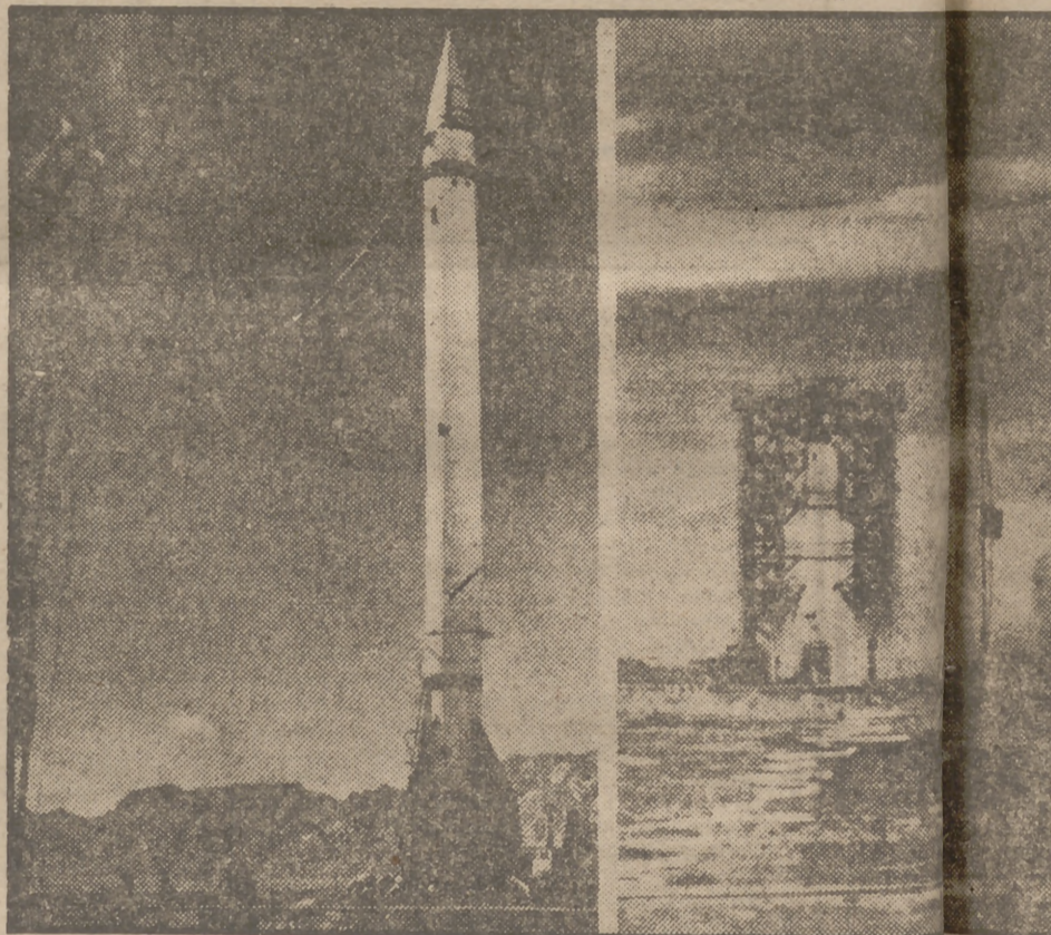
Esta es la versión americana del cohete "V-2" alemán. Es conocido como "Wiking", y fue probado hace dos años en Nuevo Méjico. En la foto de la izquierda se ve el artefacto preparado para ser disparado. La otra foto recoge el momento en que se despega de la plataforma donde estaba emplazado. El "Wiking" alcanzó una altura de 3.600 kilómetros y una velocidad de 3.600 kilómetros por hora.
