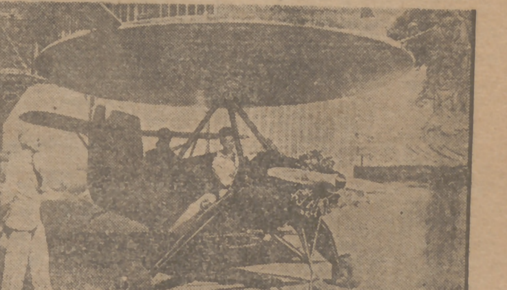
Este es el modelo 1940 de un aparato ideado por Jonathan E. Caldwell, los restos de cuyos planos han sido encontrados cerca de Glen Burnie (Maryland) por un oficial de la Aviación norteamericana, que le puso a esta especie de autogiro el nombre de "salsera voladora". (Foto A. P.)
