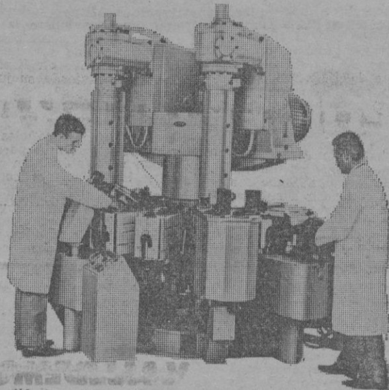
Máquina universal de moldear por extrusión la materia PVC para la producción incluso de calzado bicolor, Mod. 100355/P3
