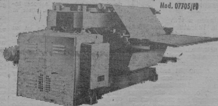
Máquina suavizadora de la superficie de cueros curtidos tipo de paso de gran rendimiento. Ancho de trabajo 1500 mm. Mod. 07705/P3
