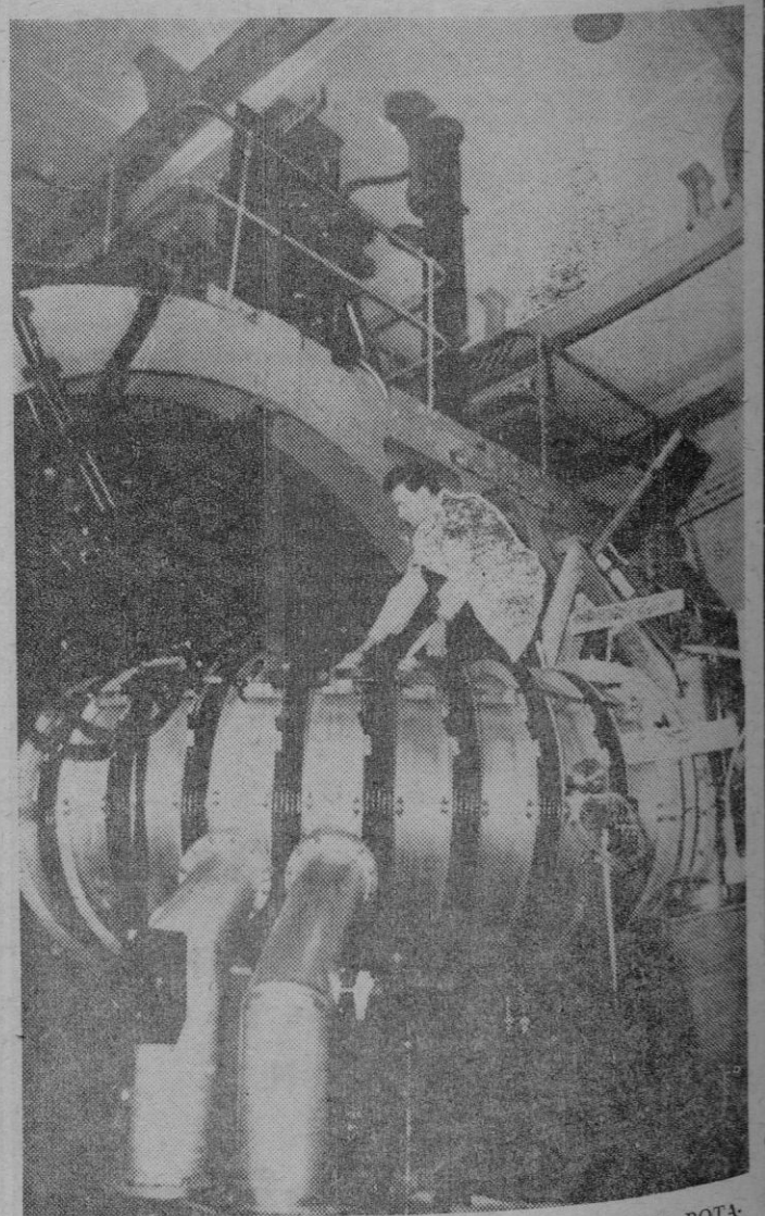
INGLATERRA. — LA AMENAZA DE ESCASEZ DE AGUA POTABLE ESTÁ YA SIENDO COMBATIDA CON EL PROGRESO DE LA ENERGIA NUCLEAR PARA USOS PACIFICOS. EN LA FOTO, UNA VISTA DE ALGUNOS DE LOS APARATOS NUCLEARES «ZETA» PARA LA OBTENCION DE HIDROGENO DEL AGUA. — (Foto CIFRA)
