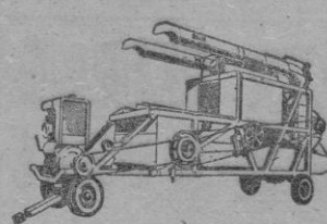
TRILLADORAS OSCA 40 CAV. Con motor gas-oil incorporado
