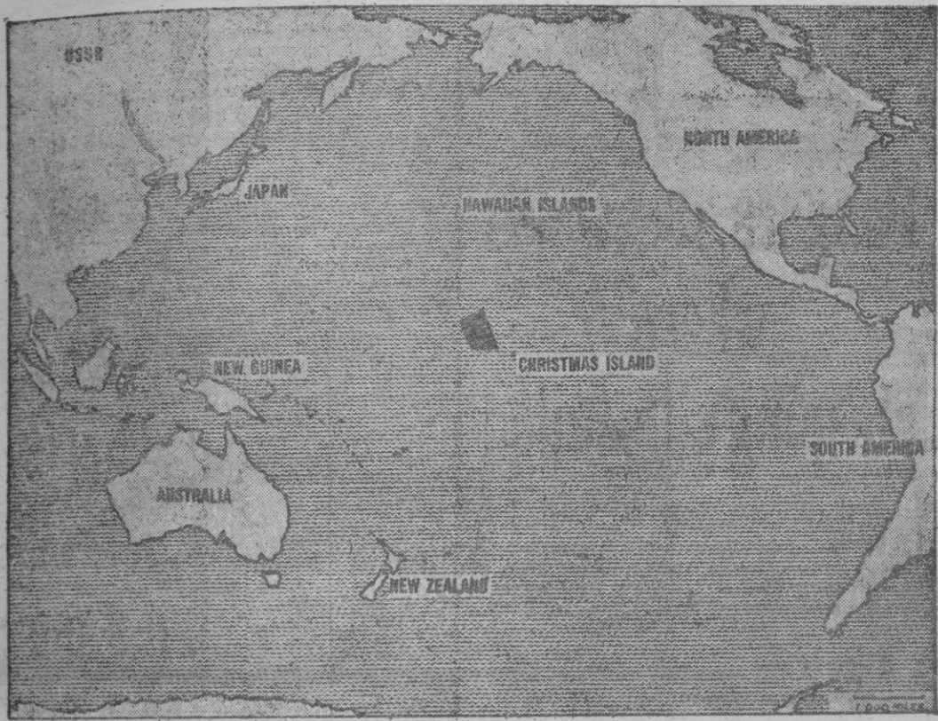
Presentamos, en el recuadro negro del centro del gráfico, en pleno océano Pacífico, la zona que los rusos se reservan para las pruebas de cohetes nucleares anunciadas para después del día 15 de los corrientes.
