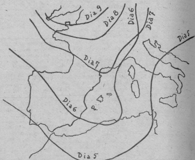
El anticiclón retrocede. Posiciones sucesivas del borde del anticiclón en las fechas señaladas en la figura. Hemos tenido que tomar como borde la isobara de 763 milímetros, ya que la presión excede de su valor normal (760 mm.) en todo el mapa.
