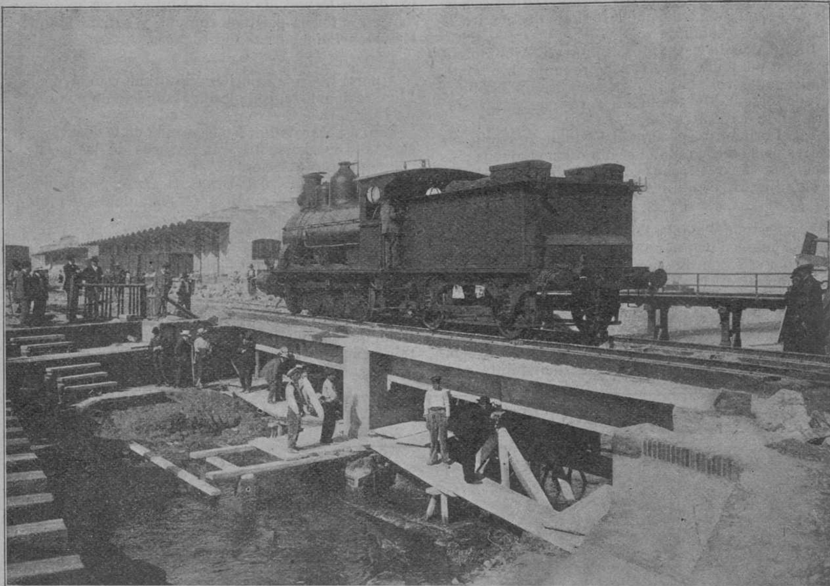
Probas, verificadas el dijous día 16, del pont de hormigón armat, construhit sobre 'l Bogatell, en la línea dels ferrocarrils de Madrit Zaragoza-Alicant.
