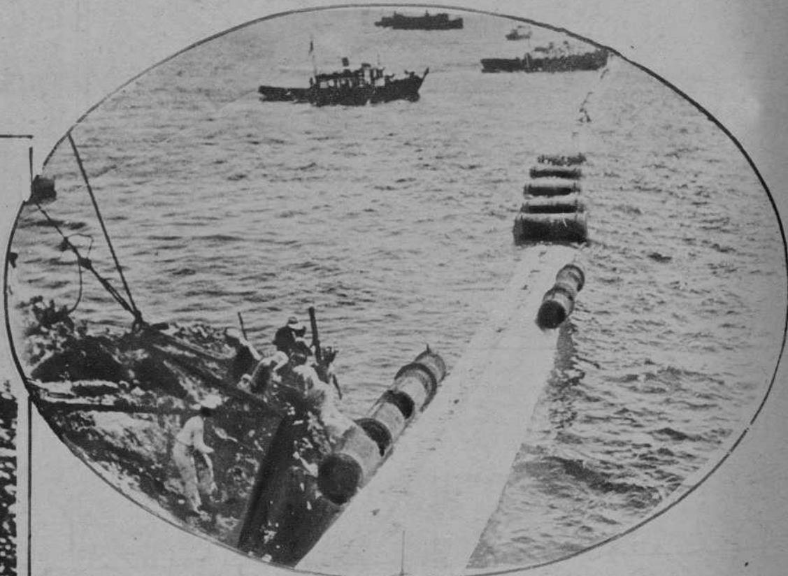
El profesor francés Georges Claude, que se propone utilizar el «gulf-stream» para la producción de electricidad. A tal efecto ha construido un tubo de dos kilómetros de longitud. Las dos primeras tentativas realizadas para obtener la inmersión del tubo, han dado por resultado la pérdida de dos tubos, cuyo coste asciende a un millón de francos. Ultimamente, la inmersión del tubo se ha llevado a cabo con el mayor éxito. Véase en la «foto» la operación de inmersión. — (Fot. Keystone)
