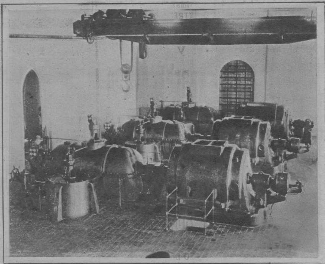
Grupo de turbinas accionadas por vapores volcánicos
