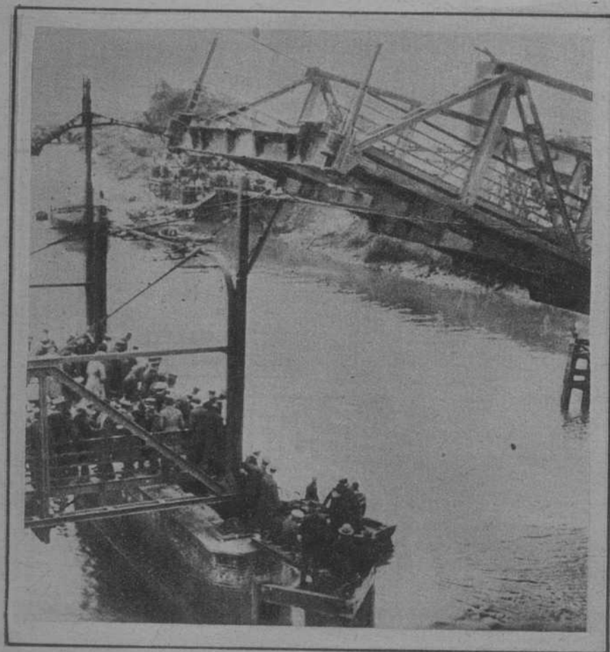
Una catástrofe en Buenos Aires.—Buscando los cadáveres de las víctimas del accidente ocurrido a un tranvía en el momento de atravesar el puente de un río, al separarse el puente para dar paso a un vapor. — (Ft. Scherl)
