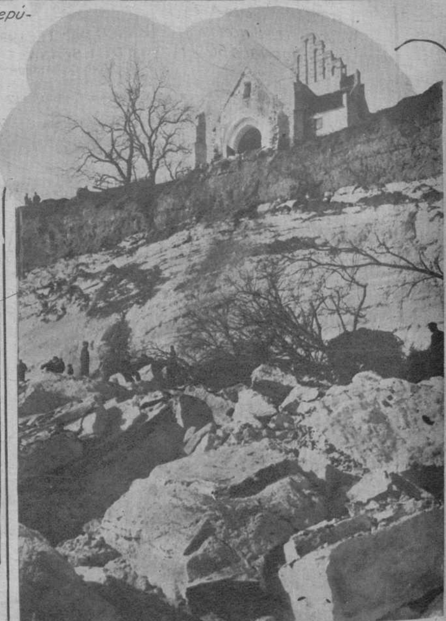
En Vinamarca, un desprendimiento de tierras ha causado grandes daños a la iglesia del pueblo de Falster. Foto Scherl
