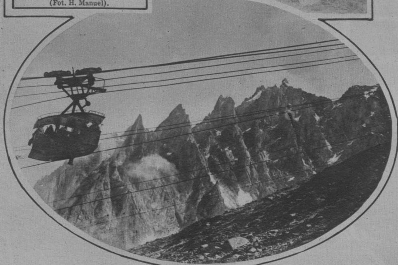
SAROYA FRANCESA.—Una vagoneta del ferrocarril aéreo que escala el Montblanch, inaugurado recientemente. Es la vía férrea más alta del mundo. (Fot. Consorcio).
