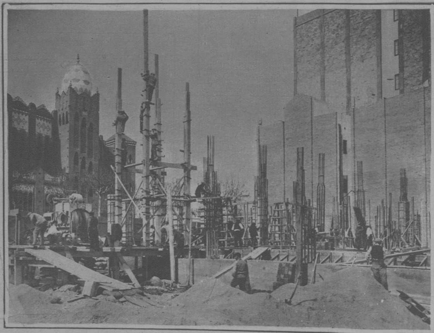
BARCELONA.—PREPARACION DE MOLDES PARA COLUMNAS DE HORMIGON EN EL EDIFICIO QUE SE CONSTRUYE EN LA CALLE DE CORTES, PARA CENTRAL AUTOMATICA DEL CLOT.
