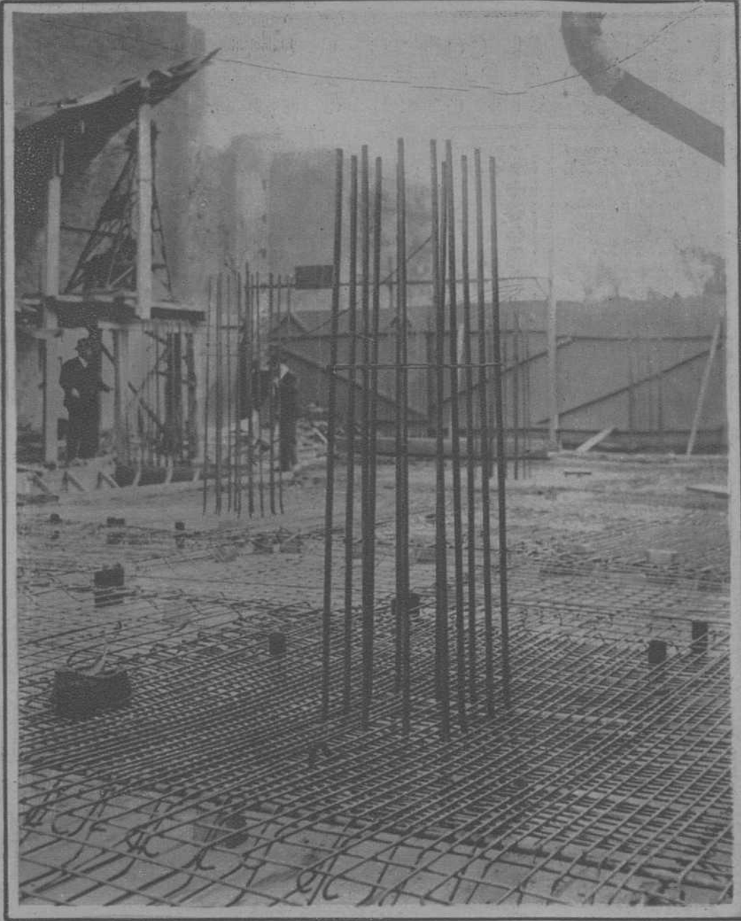
BARCELONA.—TRABAJOS DE EMPARRILLA- DO EN LA CENTRAL AUTOMÁTICA LLAMA- DA DE ARENAS, QUE SE PONDRÁ EN FUN- CIONAMIENTO JUNTAMENTE CON LAS OTRAS TRES DE BARCELONA.
