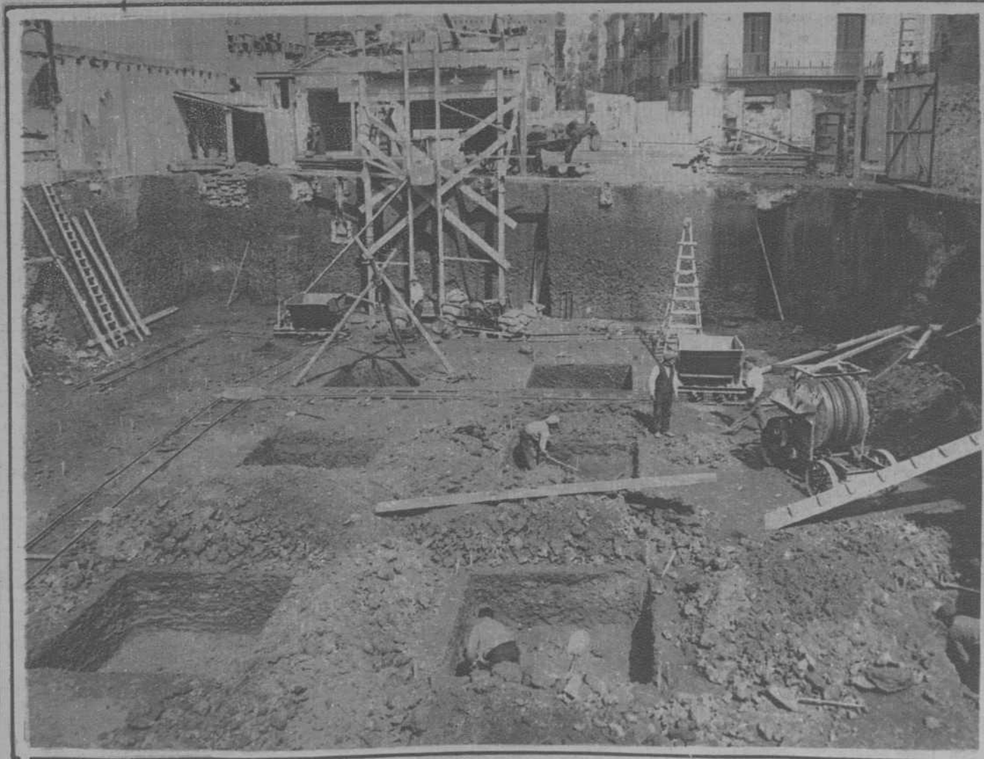
BARCELONA.—OBRAS DE CIMENTACION DE LA FUTURA CENTRAL AUTOMÁTICA DE TRAVESERA, EN LA CALLE DE SALMERÓN, ARTE- RIA CENTRAL DE LA POPULOSA BARRIADA OBRERA.
