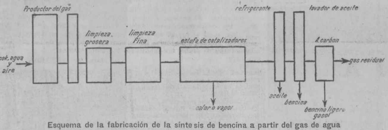
Esquema de la fabricación de la síntesis de benzina a partir del gas de agua
