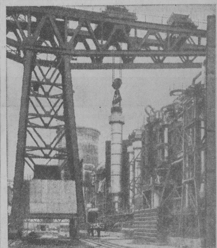
Grúa gigante, colocando un convertidor. (Fábrica de Billingham-ou-Tees.)
