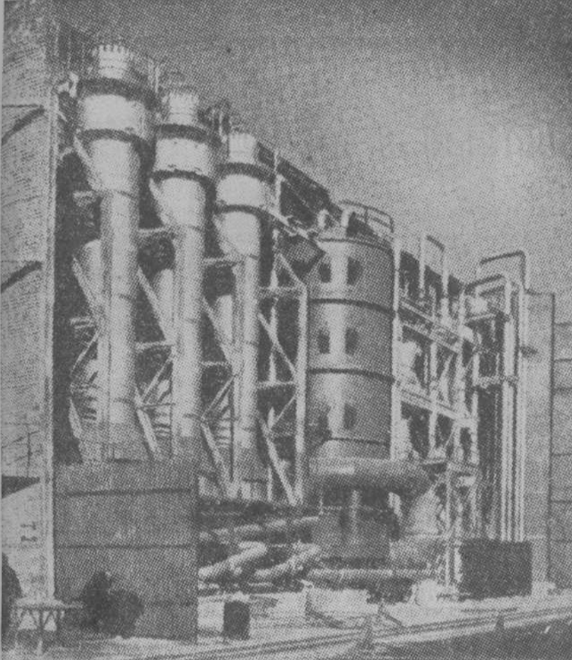
Convertidores de alta presión para hidrogenación del carbón. (Fábrica de Billingham-ou-Tees.)
