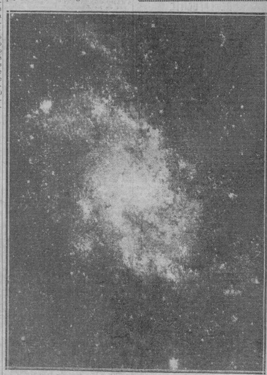
Nebulosa espiral en la constelación del triángulo. Fue obtenida la "foto" por el Observatorio del Monte Wilson y necesitó una exposición de ocho horas y treinta minutos
