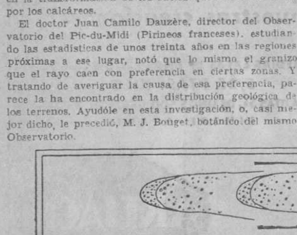
Las cintas o mangas de granizo, tales como dejan su huella sobre los campos
