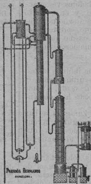
Aparato destilación continua á vapor. Producción del alcohol de 95 à 96°, ó sean 40° Cartier.
