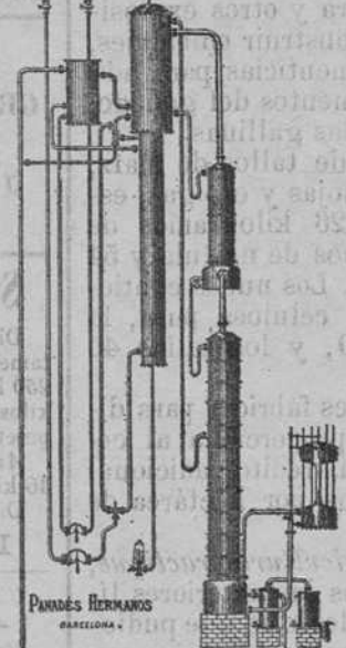
Aparato destilación continua á vapor. Producción del alcohol de 95 á 96°, ó sean 40° Cartier.
