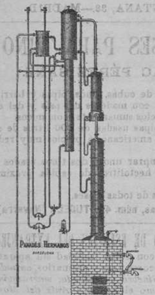
Aparato destilación continua á fuego directo. Producción del alcohol de 95 á 96°, ó sean 40° Cartier.
