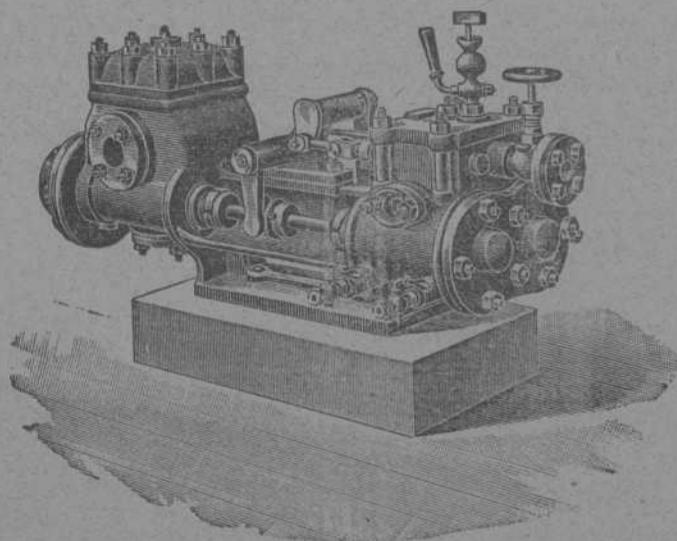
Bomba de vapor «DUPLIX»
