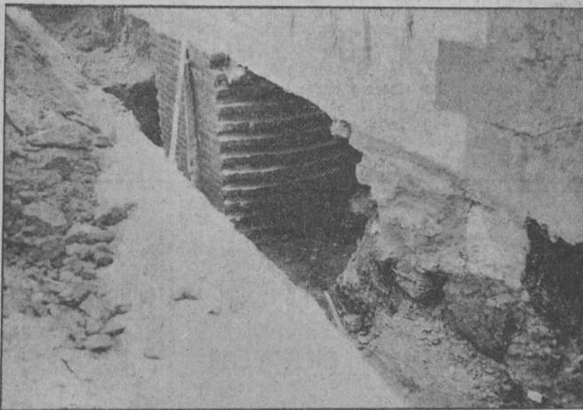
DETALLE DE LA RECONSTRUCCION DE LOS CIMIENTOS EN UN EDIFICIO DEL SANATORIO (Foto Samot.)
