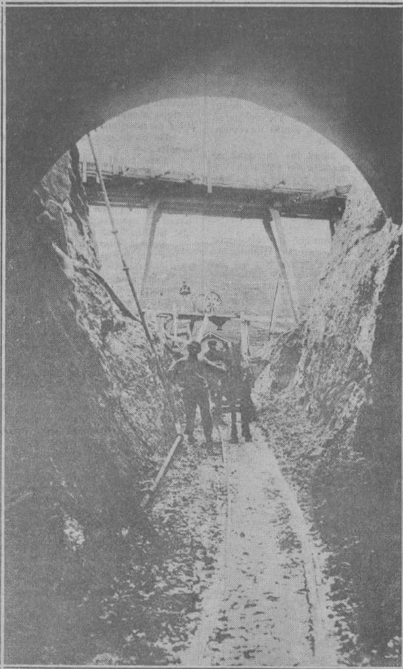
LAS OBRAS DEL PANTANO DEL EBRO.—Por esta boca de uno de los túneles de desagüe de fondo el Ebro, desviado, verterá el agua mientras se construye el dique que formará, por fin, el pantano. (Véase información en segunda plana.—Foto Alejandro.)
