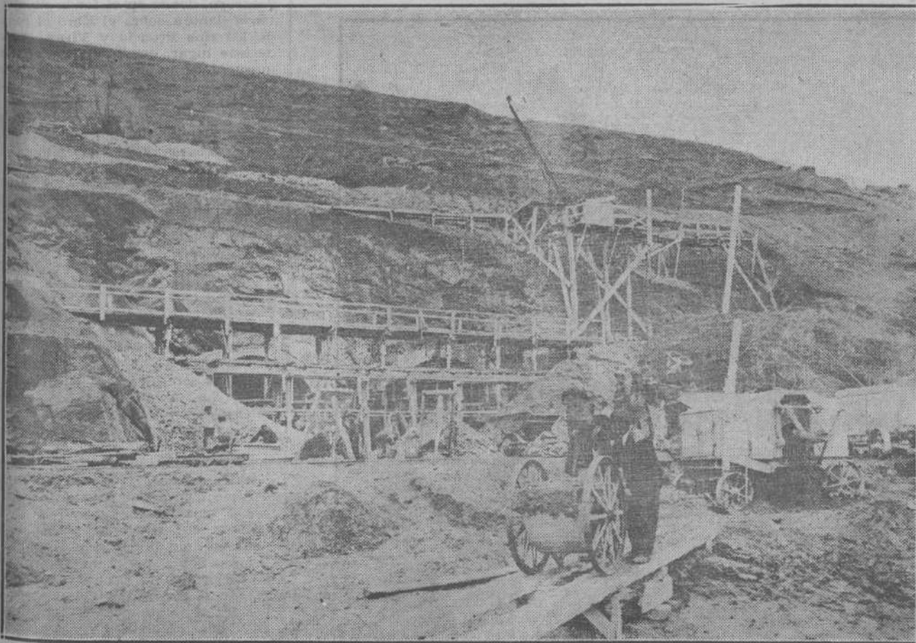
LAS OBRAS DEL PANTANO DEL EBRO.—La salida de los seis túneles que componen la base de la gran obra hidráulica.—En primer término, las hormigoneras preparan las masas de cemento que han de revestir las paredes de los túneles. (Véase la información en segunda plana.—Foto Alejandro.)
