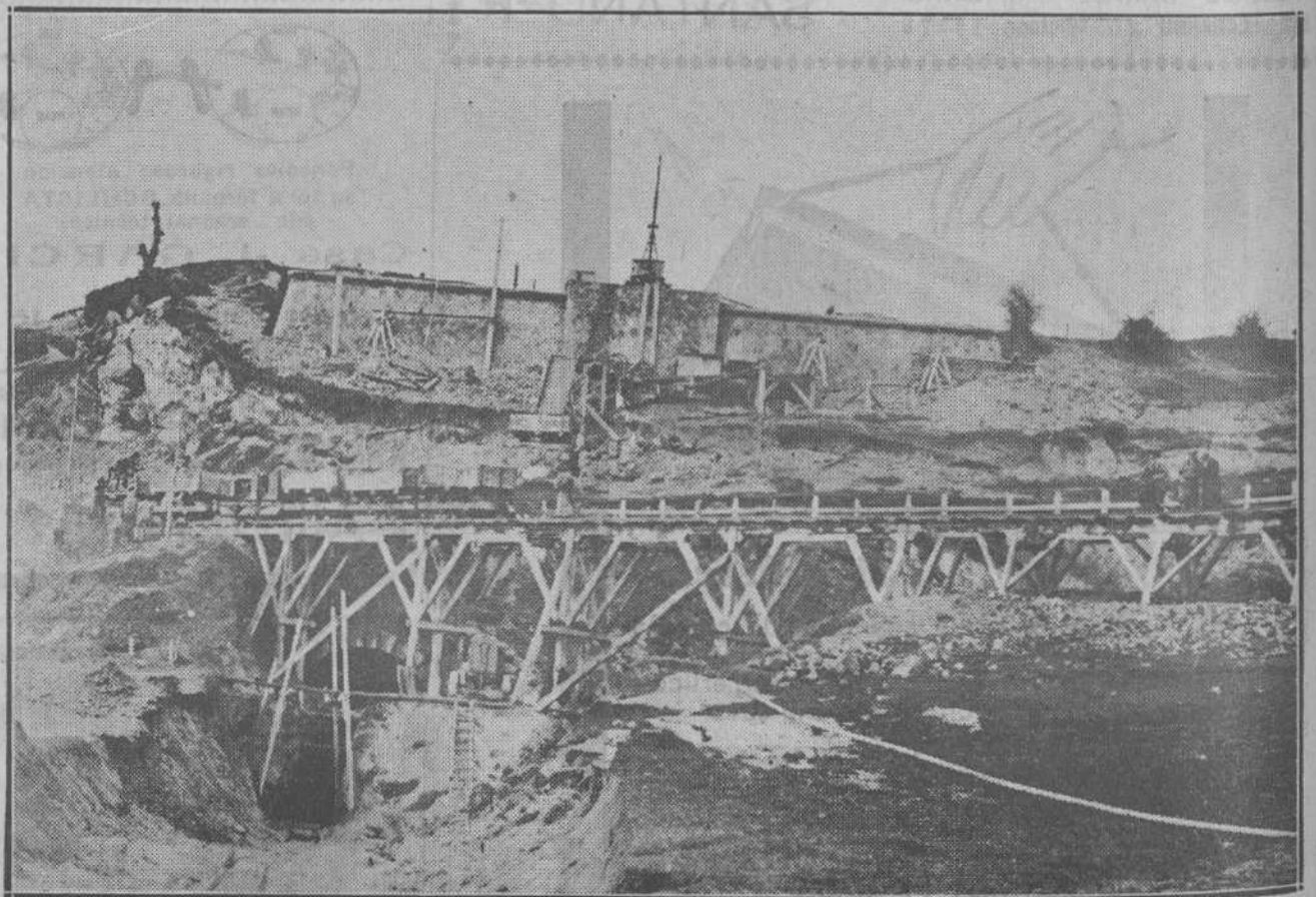
LAS OBRAS DEL PANTANO DEL EBRO.—Detalle interesante de la entrada de los túneles de fondo, por donde será desviado el río. Las obras en este lugar van muy adelantadas. En la parte superior de la foto, sobre la manpostería se advierte el lugar donde será colocada una de las casetas de compuertas. (Véase la información en segunda plana.—Foto Alejandro.)
