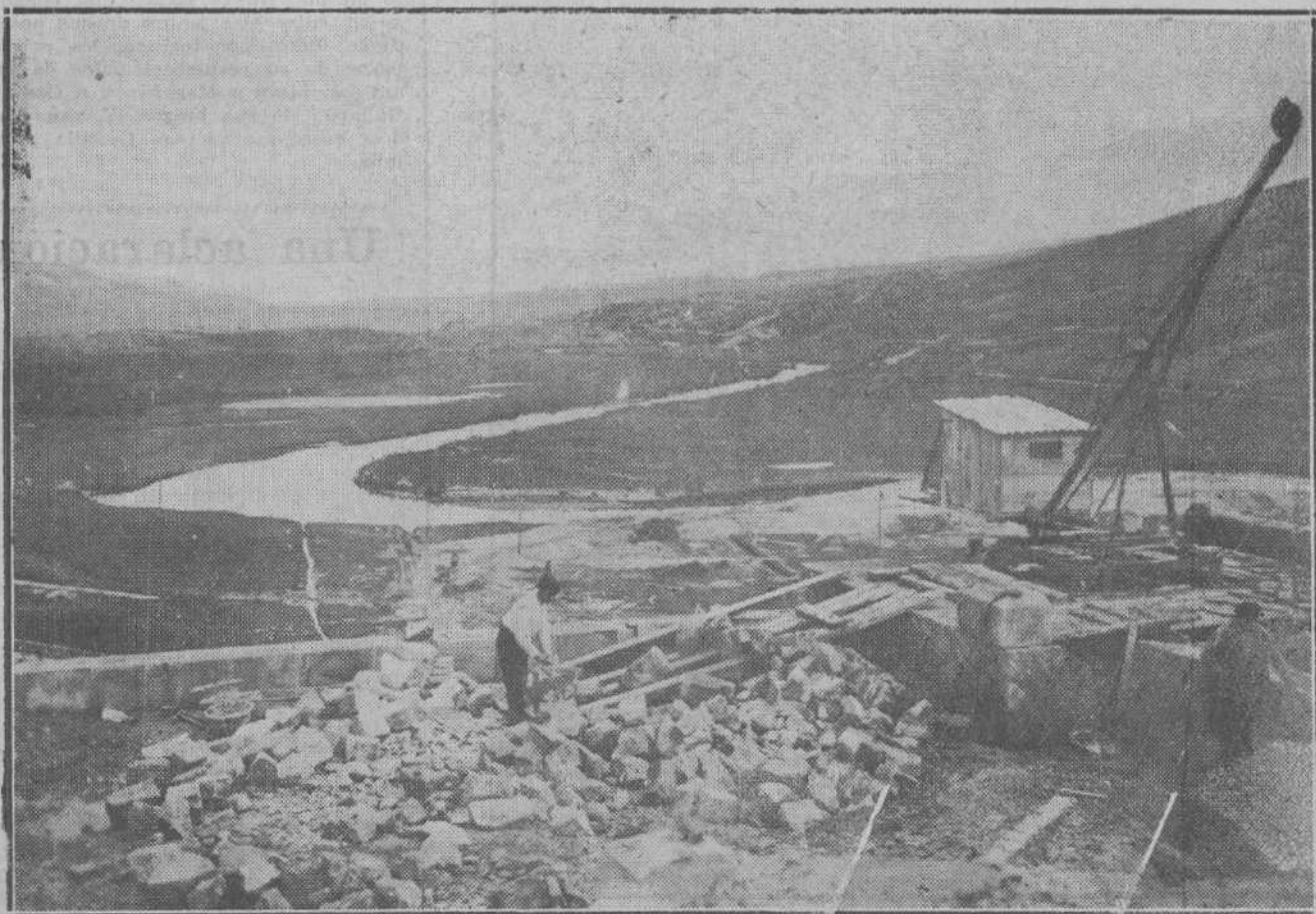
Desde lo alto de una de las entradas de los túneles de fondo, Alejandro obtuvo esta fotografía del lugar exacto donde será desviado el río.
