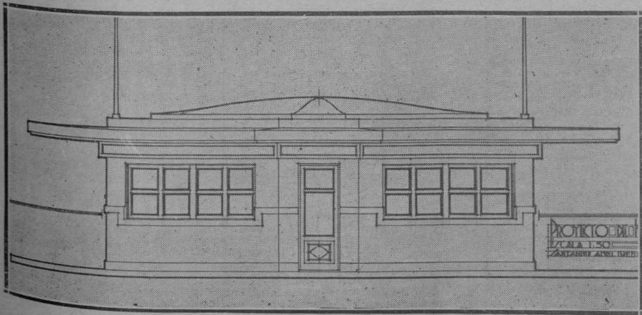
Disposición de una de las secciones del gran kiosco que será construido en la Avenida de las Estaciones.
