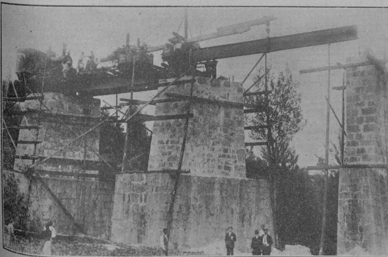
CASTRO URDIALES.—Las obras del viaducto de Dombergón, del ferrocarril minero Castro-Alen. Colocación de una viga metálica de once y medio metros. (Foto de la Torre).
