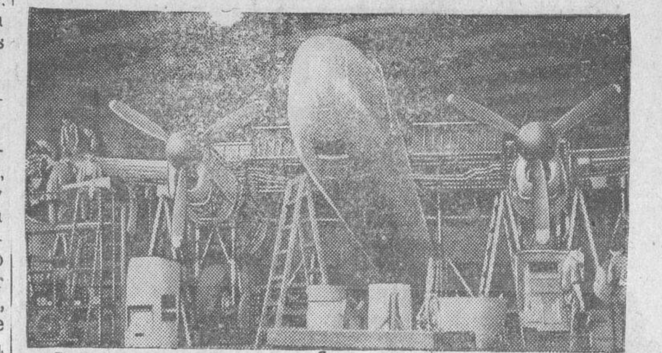
Este aparato "Lancastrian", lleva dos motores de propulsión por reacción y otros dos de émbolo, tipo "Merlin". Cuando vuele, será el mayor avión de tipo pesado movido por reacción. (Foto Calpe).
