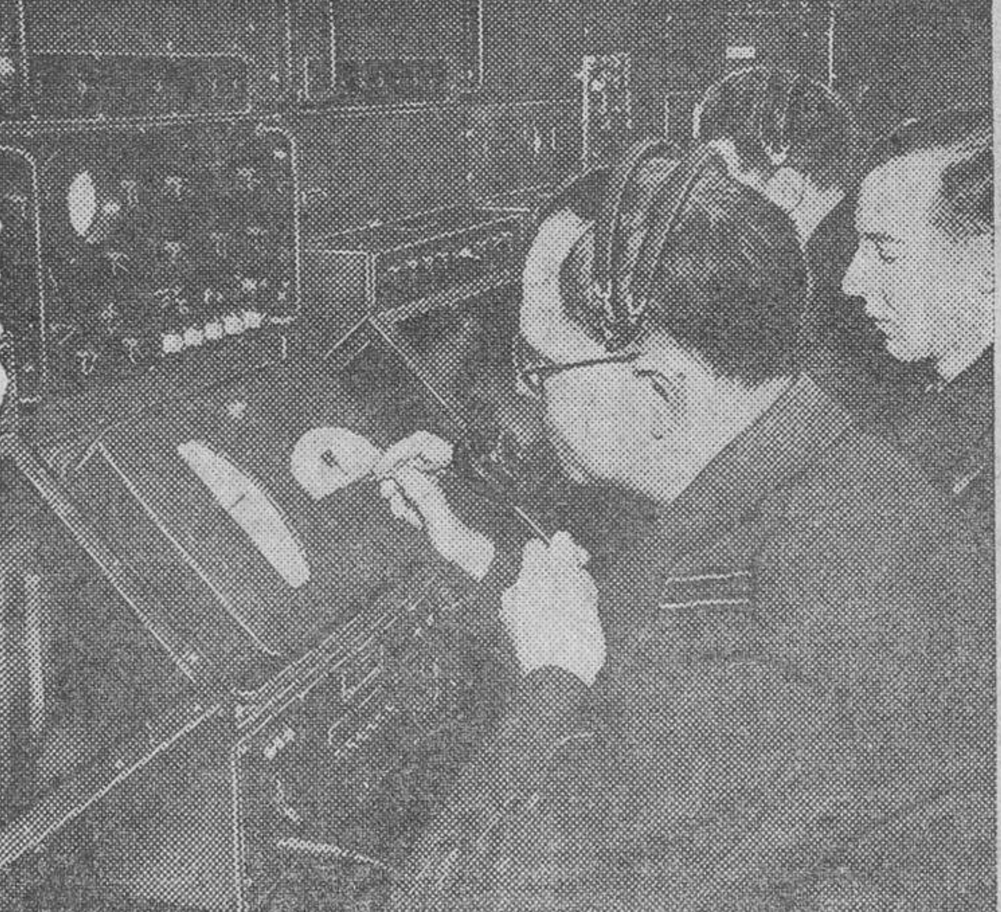
Vista interior de una estación «radar», tipo GCA, con los operadores en la mesa de control.
