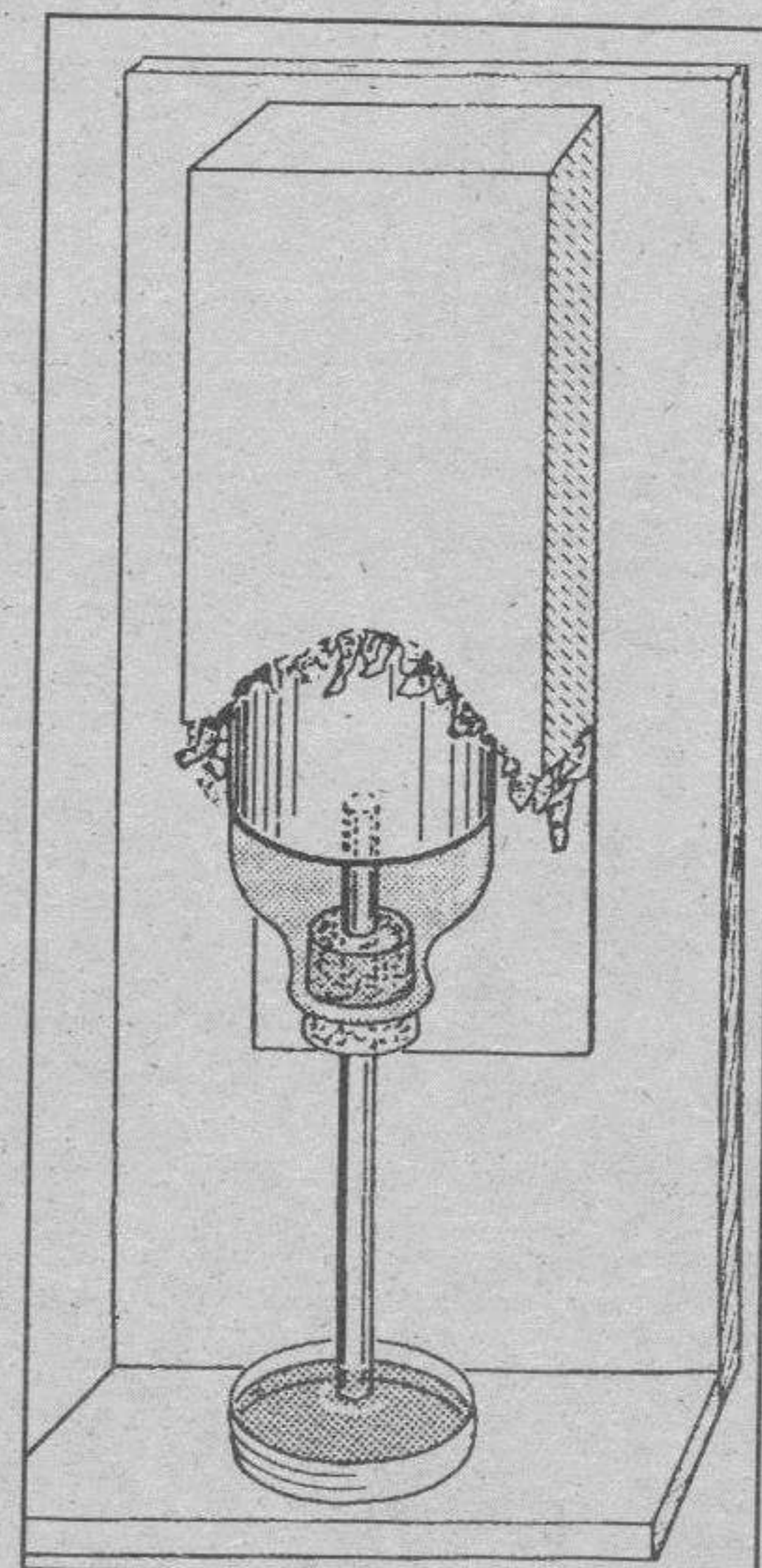
Barómetro
