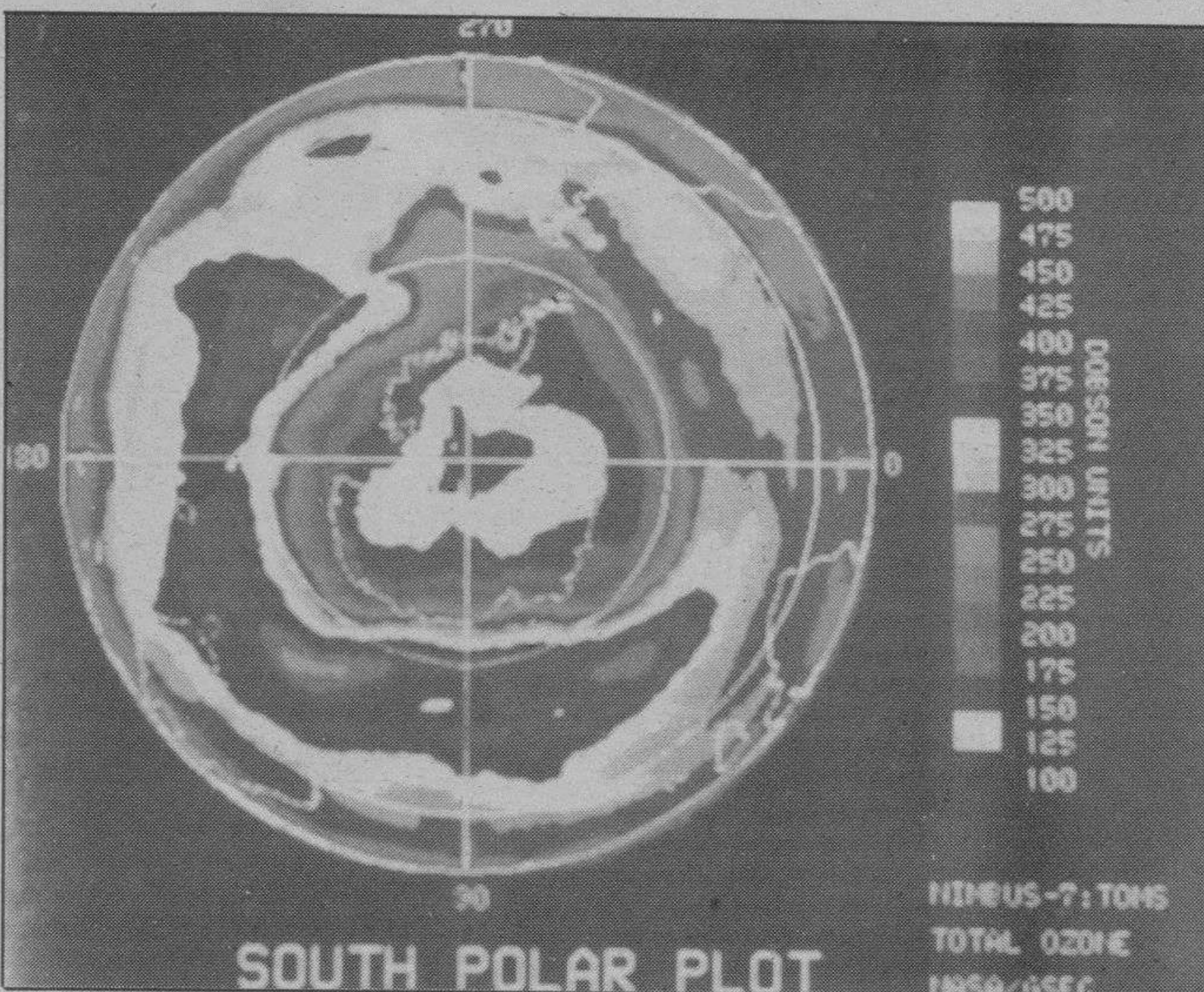
El satélite Nimbus, utilizando la técnica de «color falso», interpretaba los datos de ordenador que señalaban el temido «agujero» de ozono en el Polo Sur. Foto Salaber/Flash Press.
