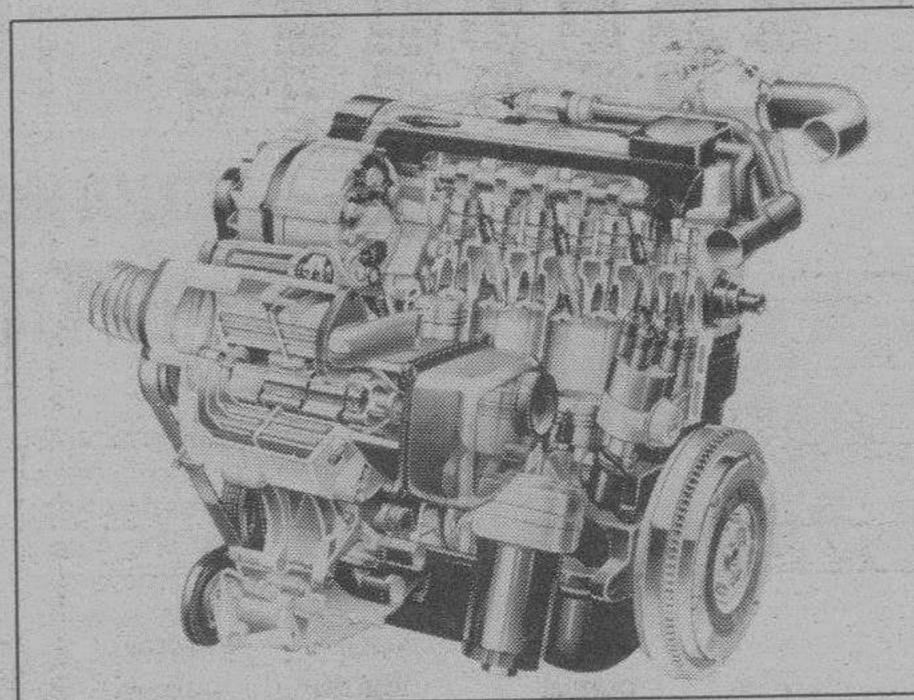
El motor incorpora el compresor «G»
