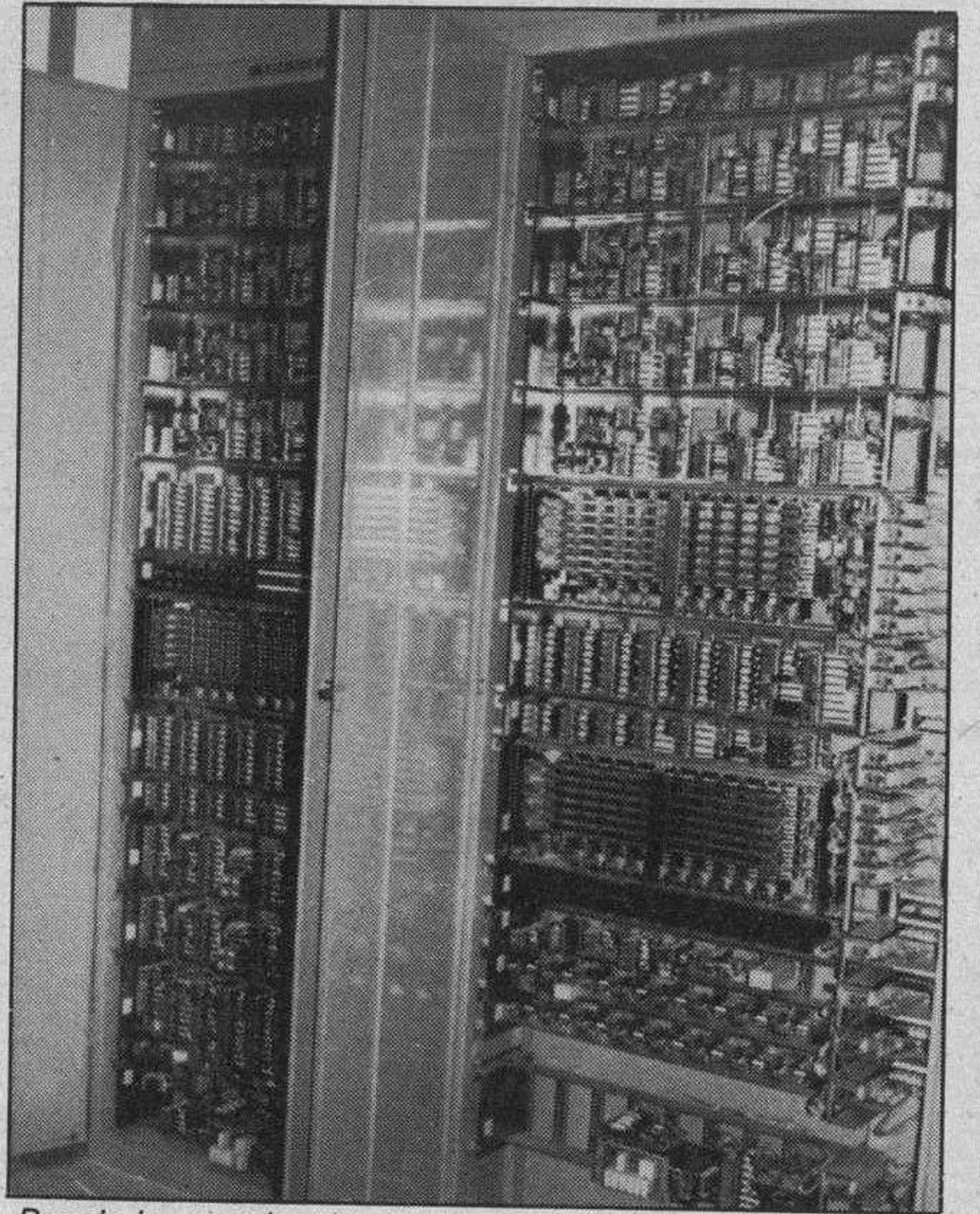
Dos de los paneles de circuitos de la central radiotelefónica.
