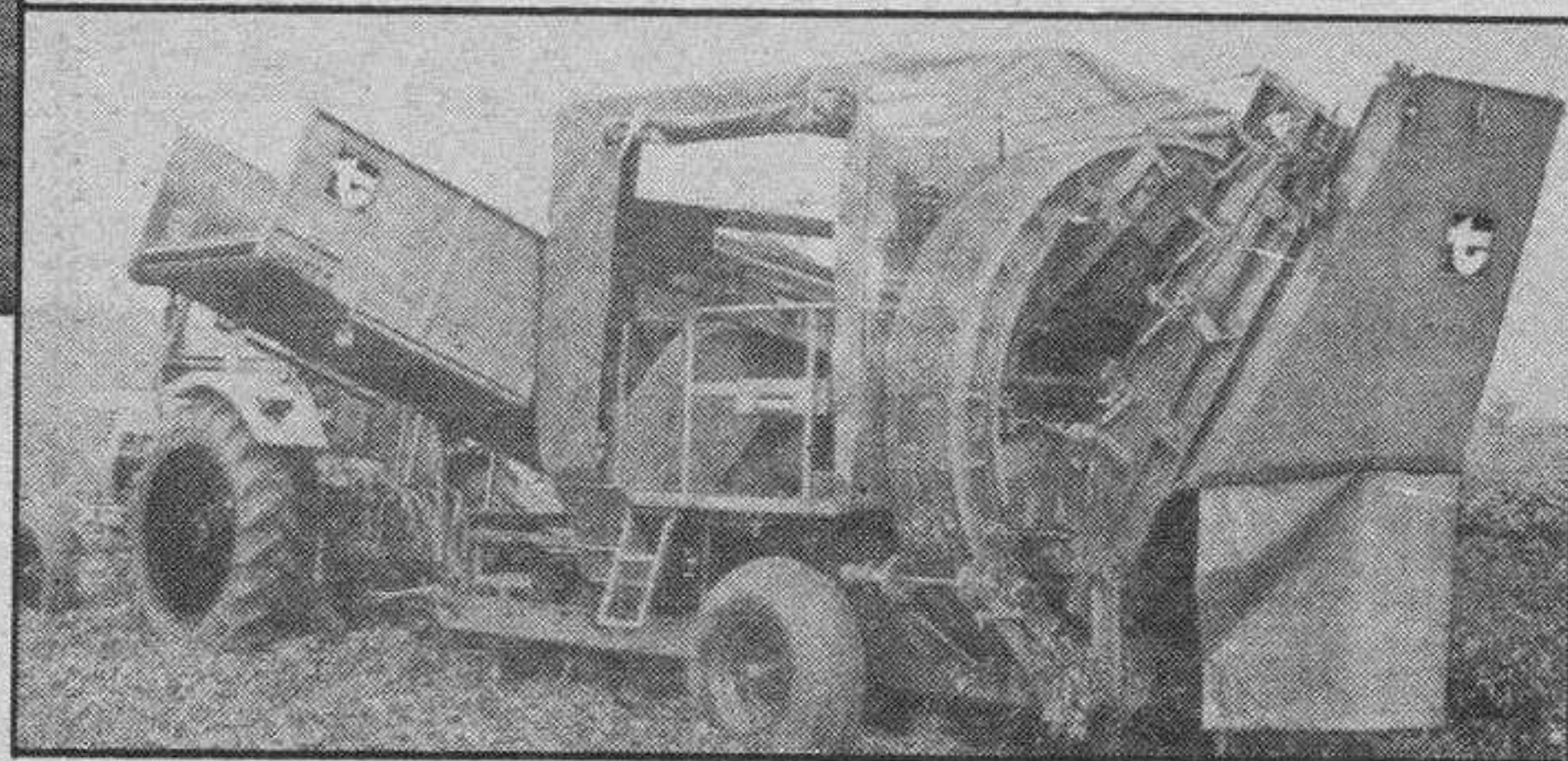
Cosechadora integral de patatas
