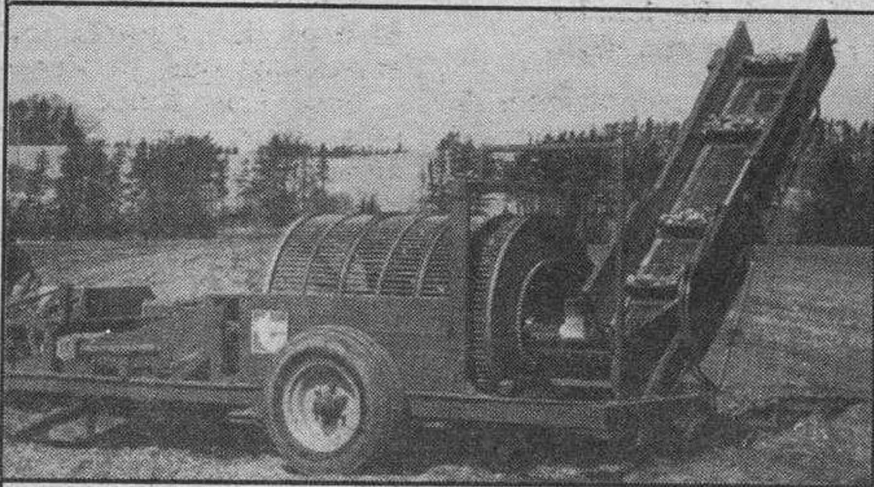
Recogedora-cargadora de piedras-N.º 1 en Europa
