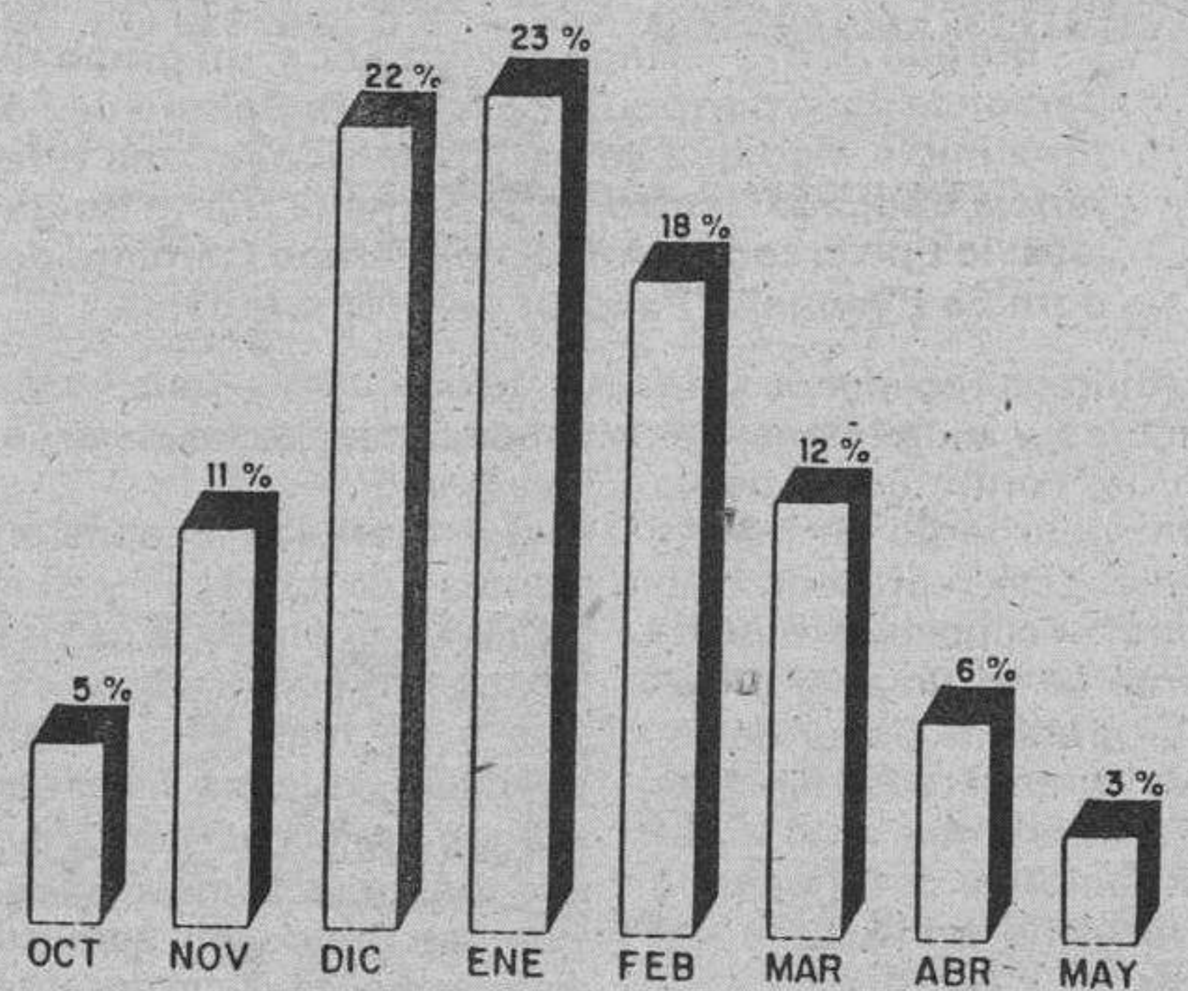
Reparto porcentual del consumo anual de calefacción.
