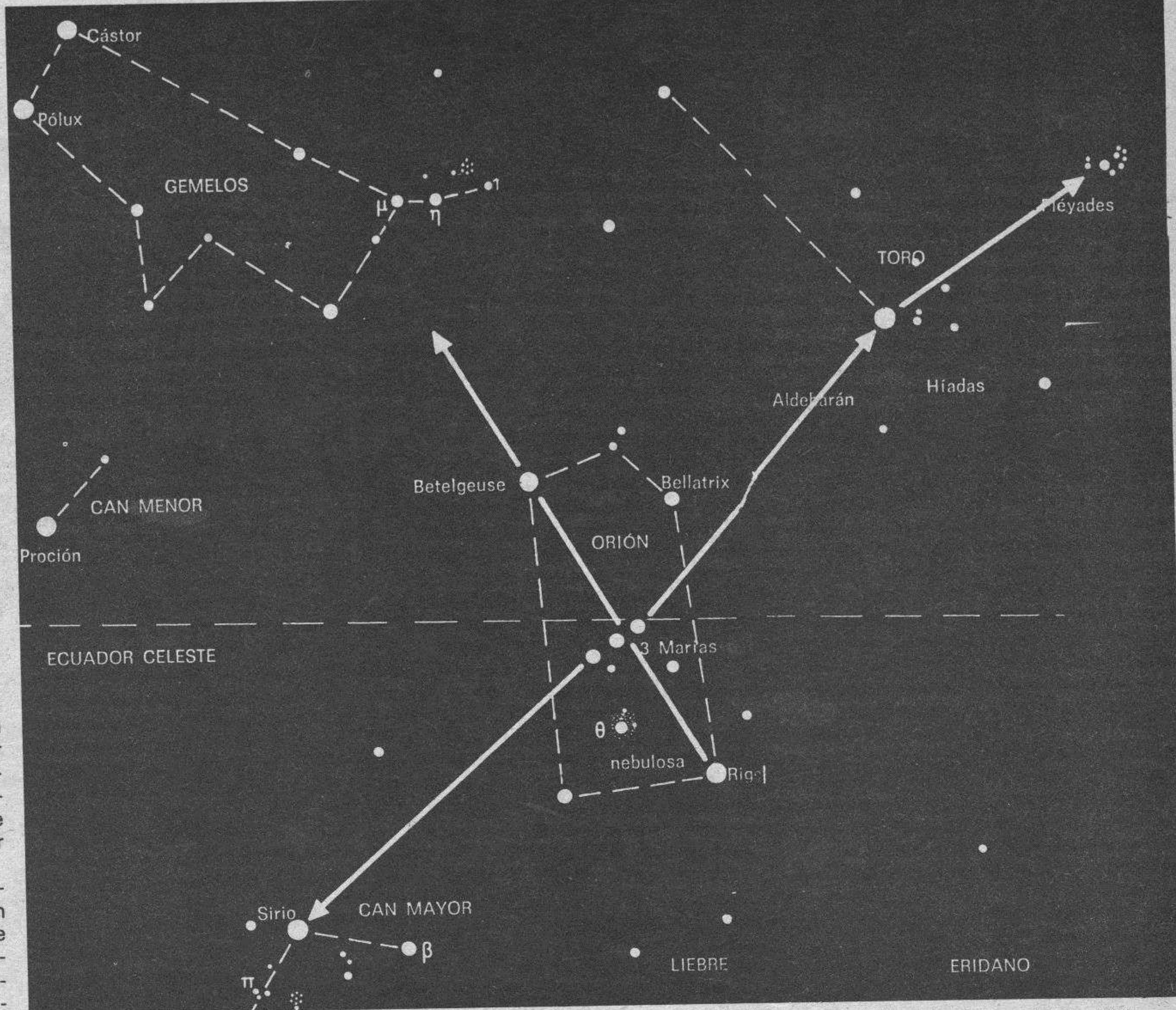
El cielo de invierno con la constelación-referencia de Orión. Obsérvense las Tres Marías alineadas en el centro del cuadrilátero. Una alineación permite encontrar los Gemelos a partir de la línea Rigel-Betelgeuse. Otra alineación, basada en las Tres Marías, va a Sirio, en el Can Mayor. En dirección contraria: Aldebarán, Híadas y Pléyades.
