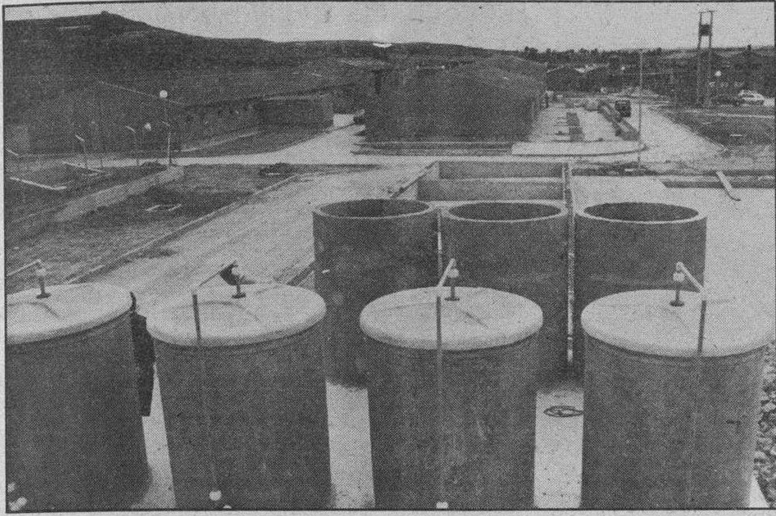
En primer término, los depósitos de tratamiento de estiércol para producir electricidad en Albillos.
