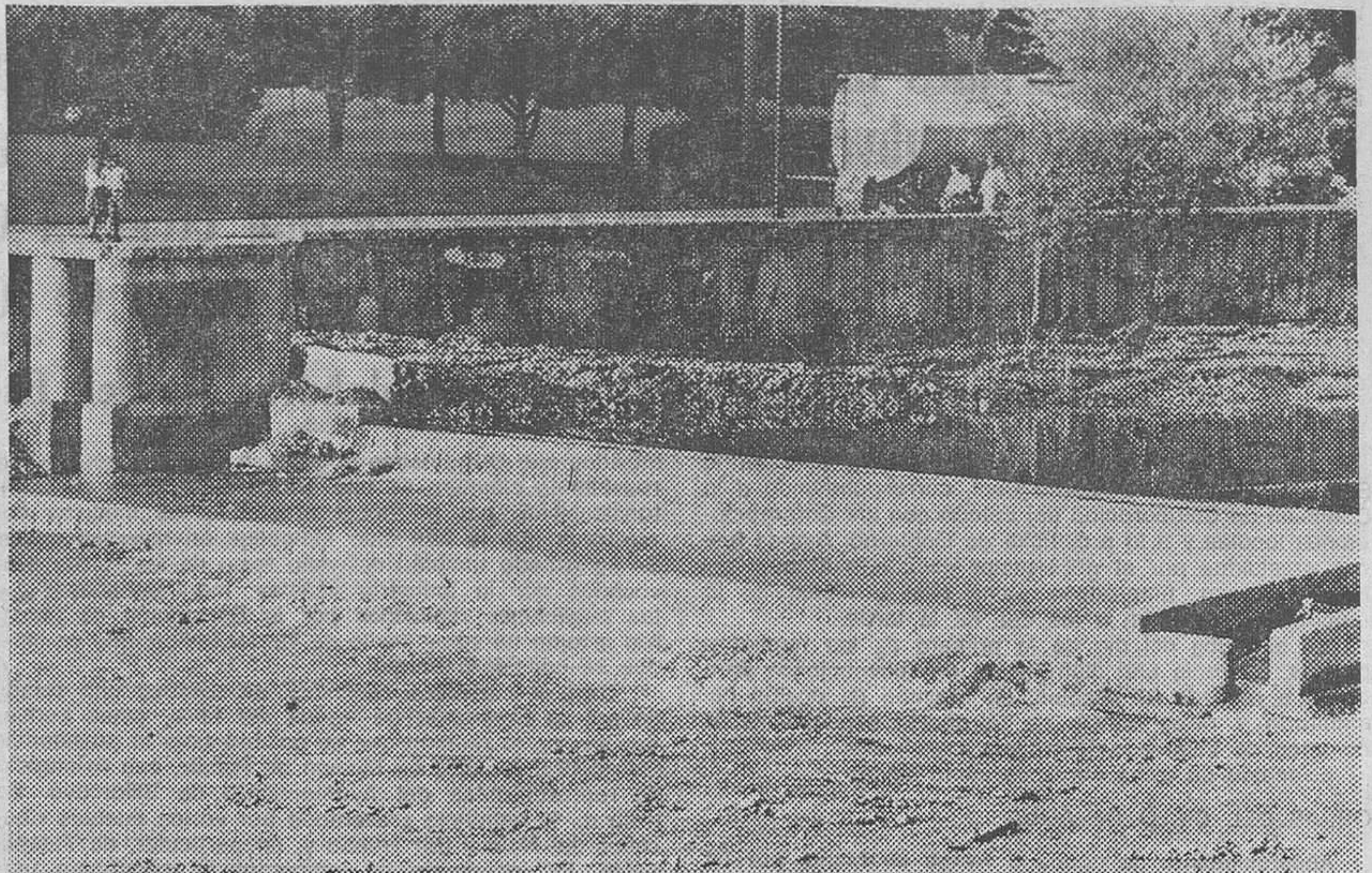
Esta es la sección reconstruida de la presa de «Los Trampones» en el río Arlanzón, frente al parque de la plaza de Logroño. Los trabajos han sido ejecutados por personal de la brigadilla municipal de obras a la vista de la extrema urgencia de esa reconstrucción que aconsejaba el estado ruinoso de la presa. — (Foto FEDE).
