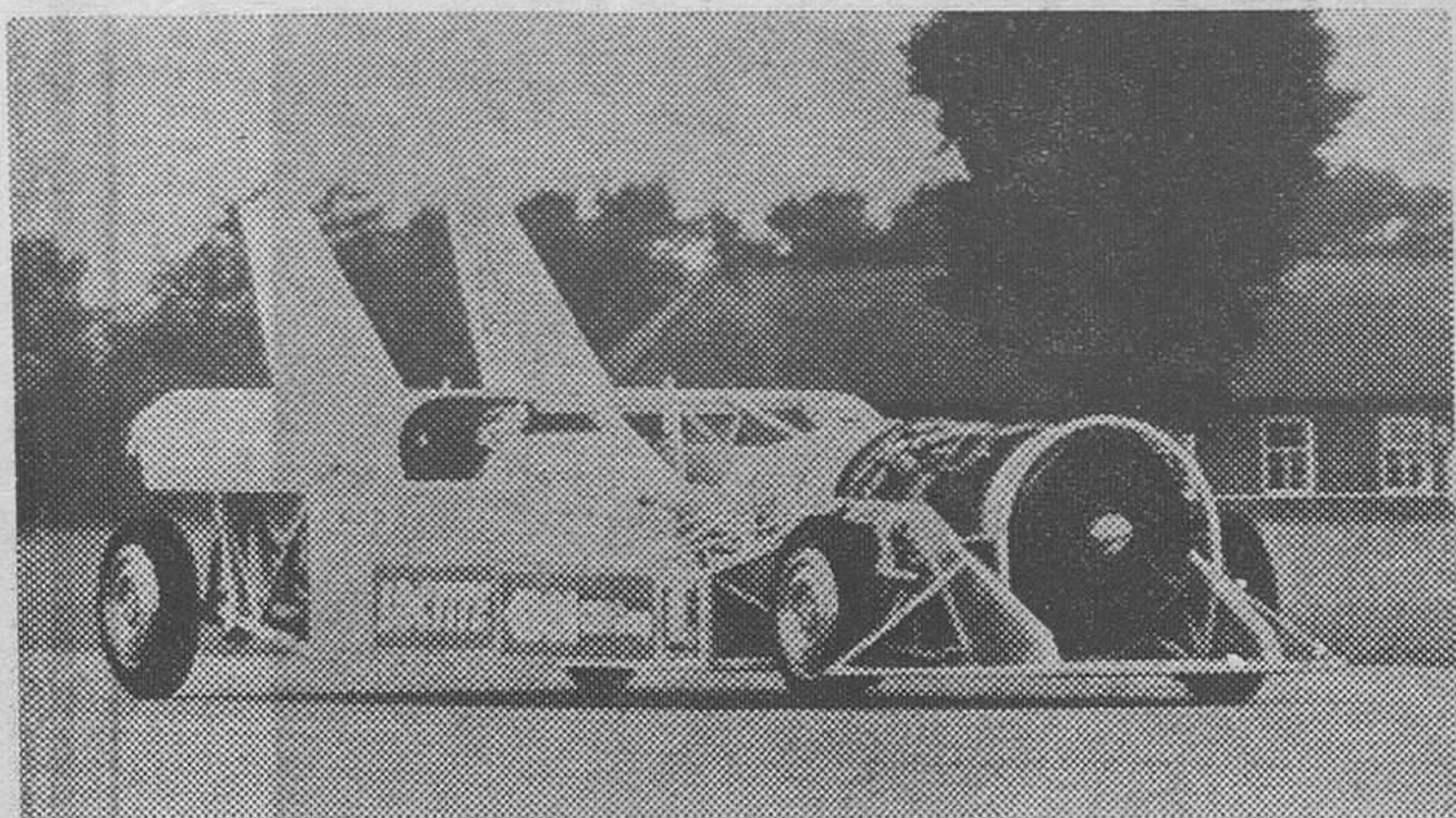
Greenham (Inglaterra). — El «Thrust 11», este «jet car», diseñado por Richard Noble, y totalmente de fabricación británica, realiza unas pruebas de velocidad en el aeródromo de las Reales Fuerzas Aéreas de Greenham. Esta máquina ha sido construida para conseguir una velocidad de más de mil kilómetros a la hora. Con ella cualquiera puede batir un record. — (Telefoto EFE-AP).
