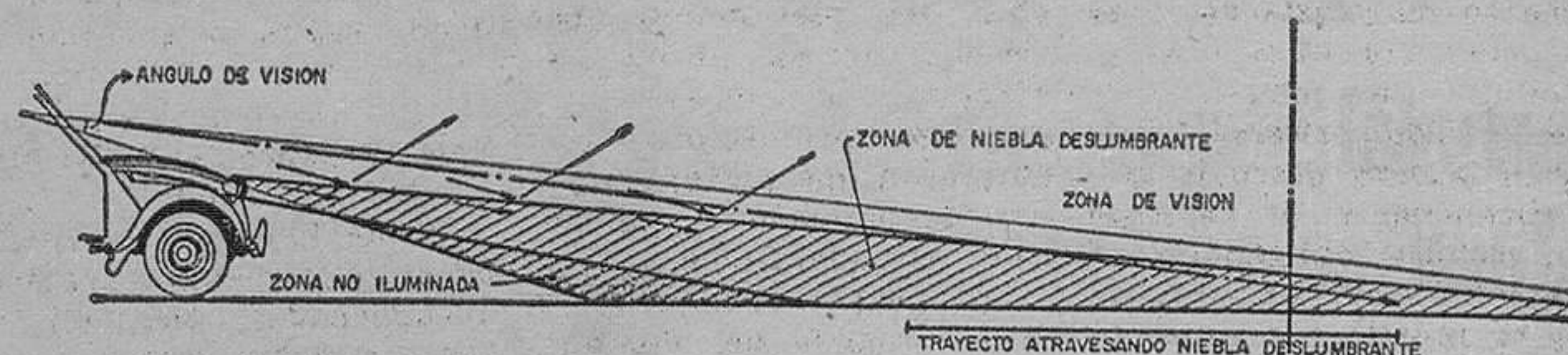
FIG. 2 FAROS CRUCE SITUADOS ALTO
