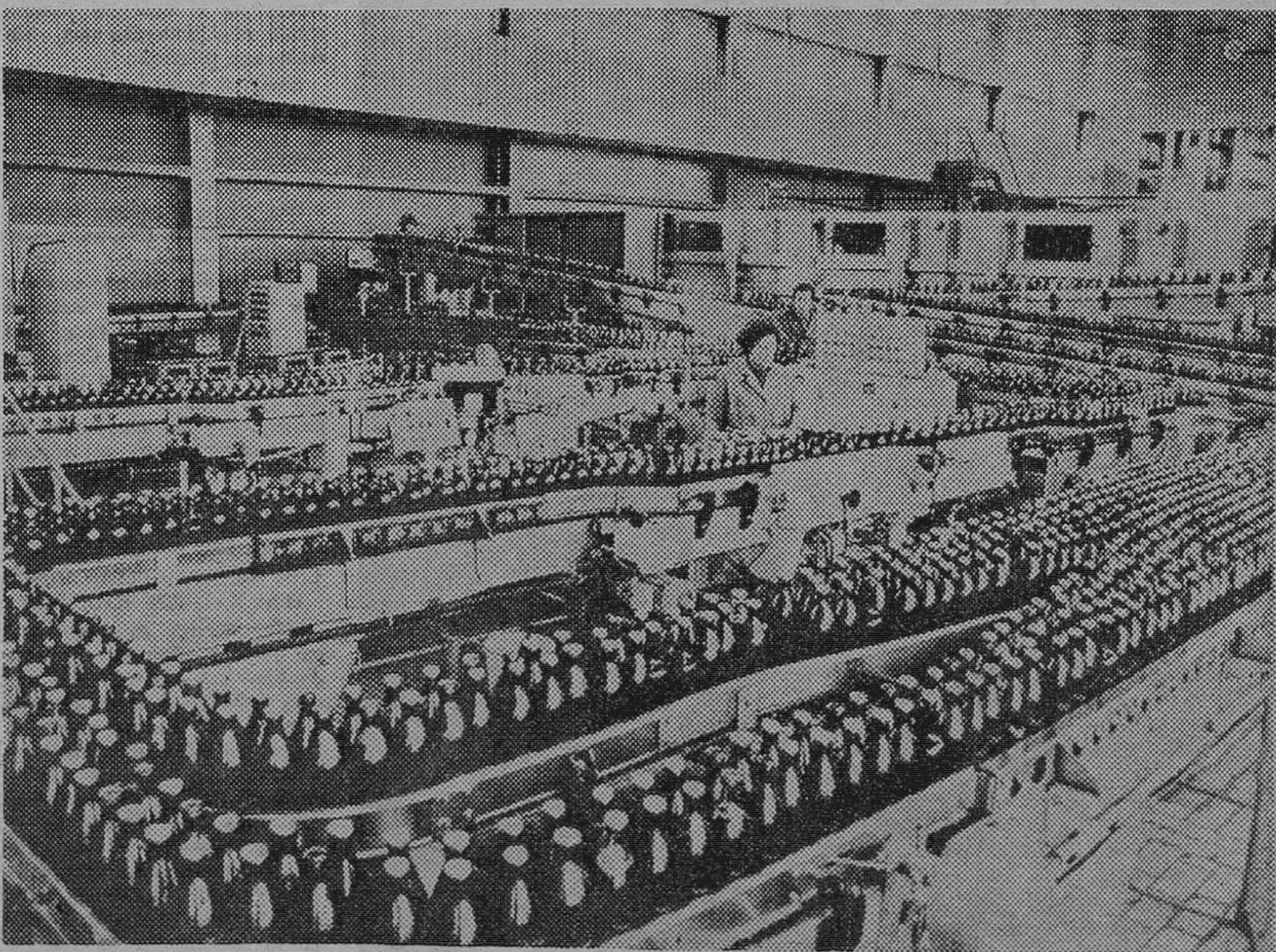
Berlin. La República Democrática alemana trata de aumentar y mejorar su producción de cerveza. Las principales instalaciones de Leipzig trabajan a ritmo acelerado y este aumento y mejora puede conseguirse gracias a dos nuevas instalaciones de embotellamiento. La República Democrática Alemana ocupa el séptimo lugar en el consumo per cápita de cerveza en el Mundo, con 106,5 litros. — (Foto FIELADN).
