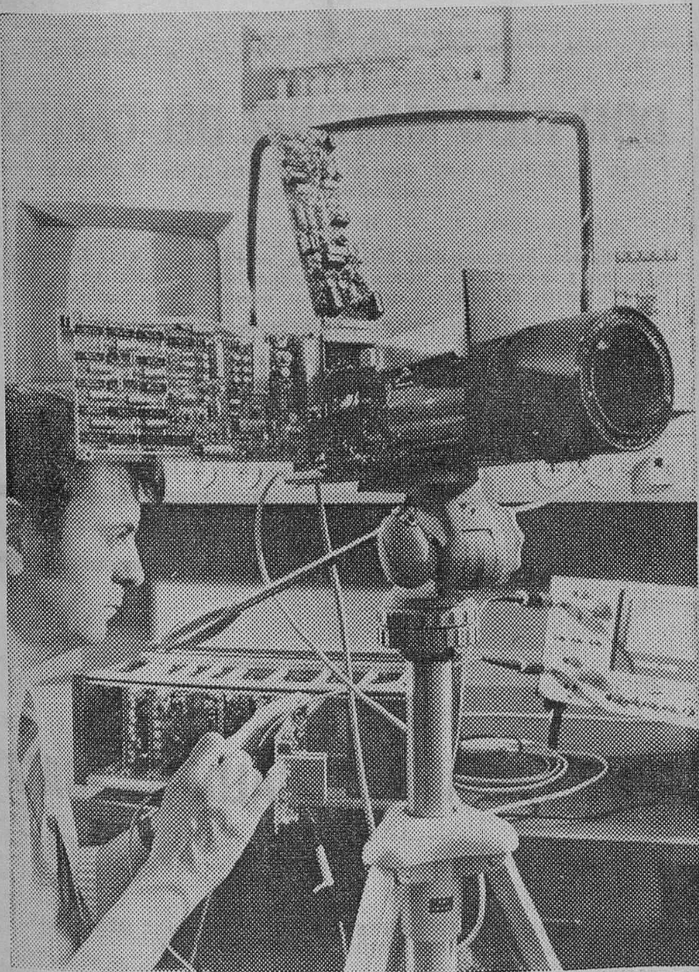
La foto muestra la nueva cámara de TV en color con un solo tubo, que en vez de precisar tres tubos para el rojo, el verde y el azul, va equipada con uno sólo, lo que permite reducir considerablemente el tamaño de la cámara. El «secreto» de esta nueva cámara, ideada por Siemens, ideal para las instalaciones móviles de color para reportajes, es un filtro de color que descompone ópticamente los tres colores fundamentales de la imagen procedente del objetivo. — (Foto FIEL).
