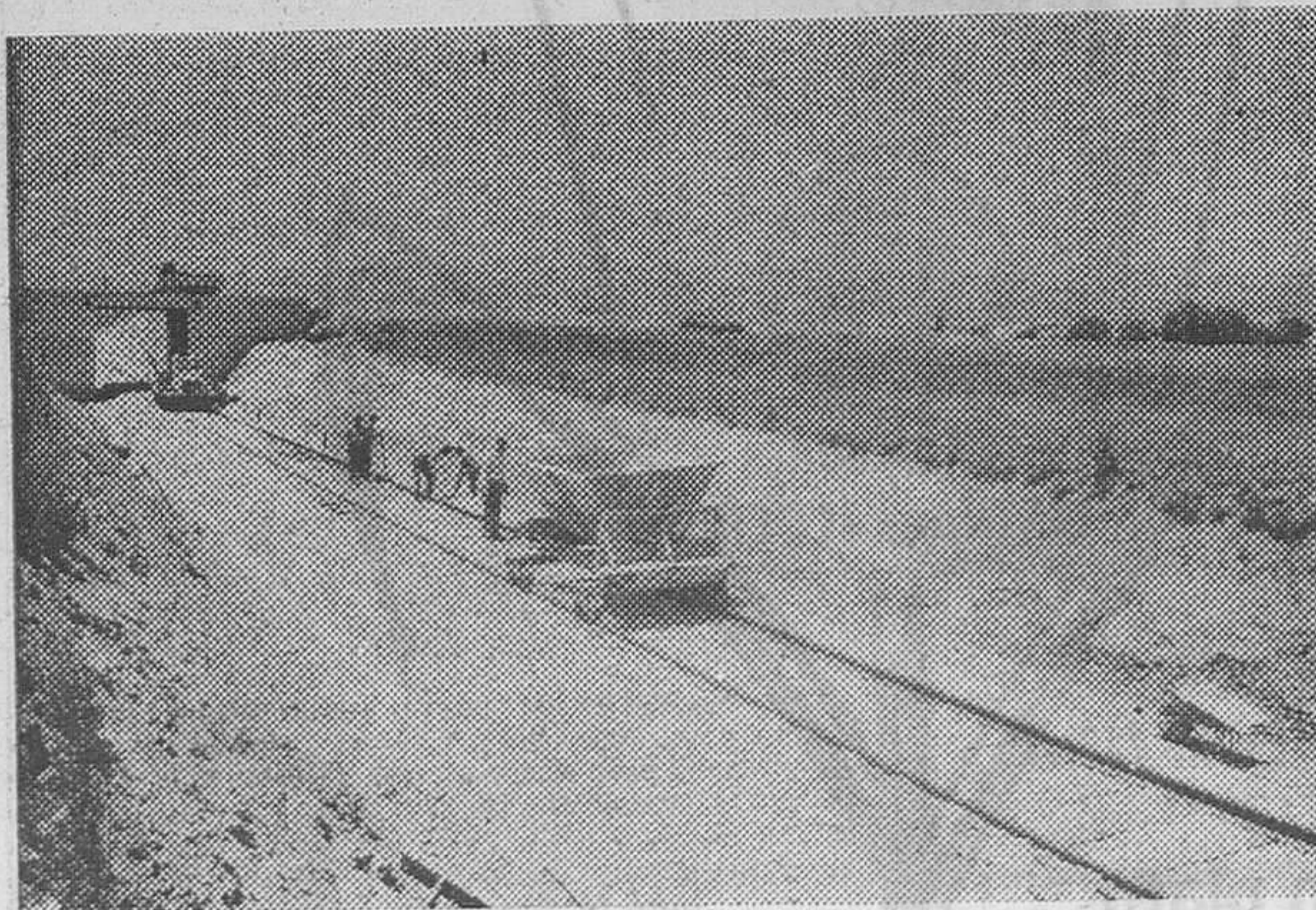
Tendido de vías para el ramal ferroviario del polígono industrial de Villalonquéjar.
