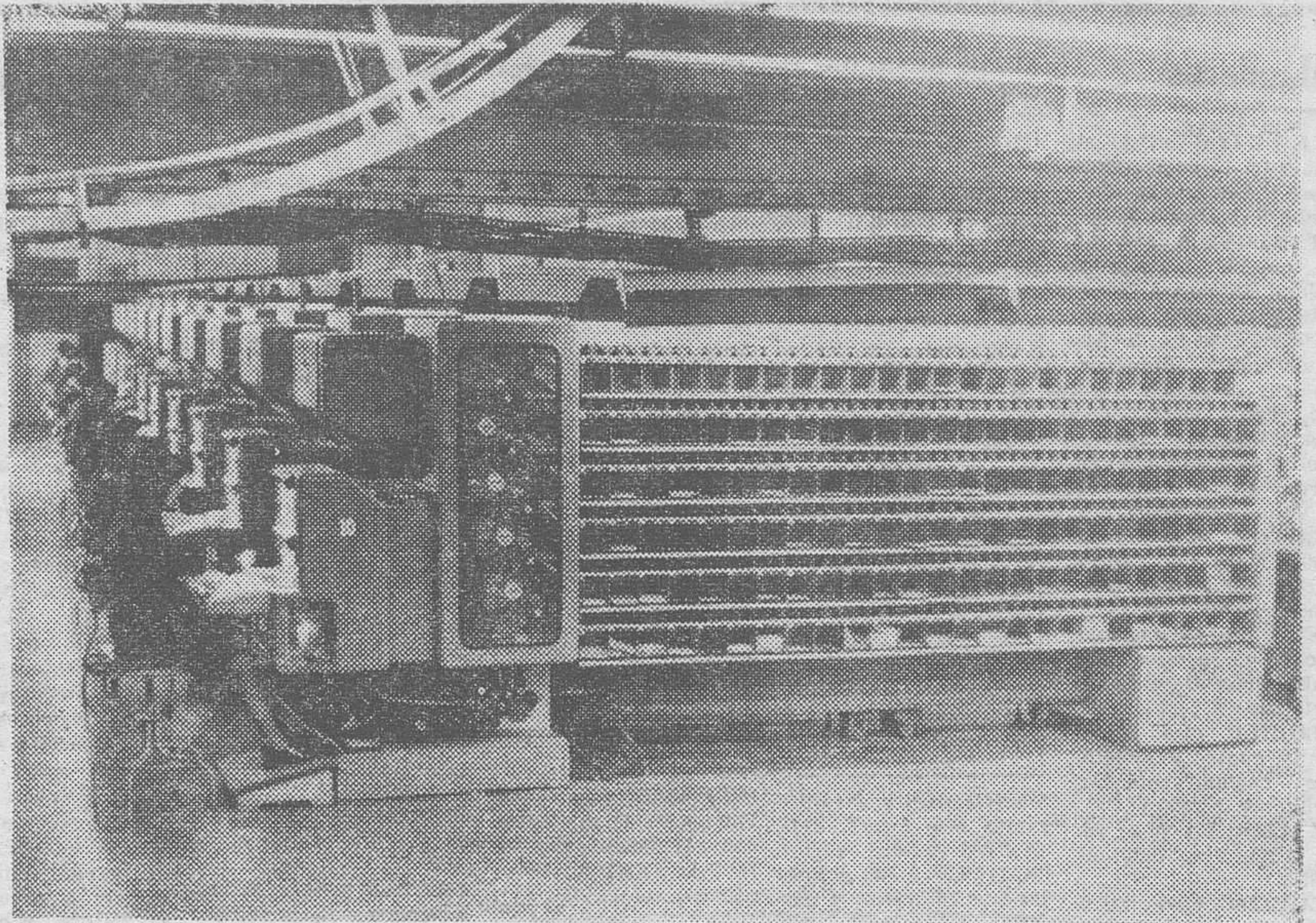
Máquinas clasificadoras «Trhissell» capaces de enviar 6.000 cartas a 144 países diferentes.
