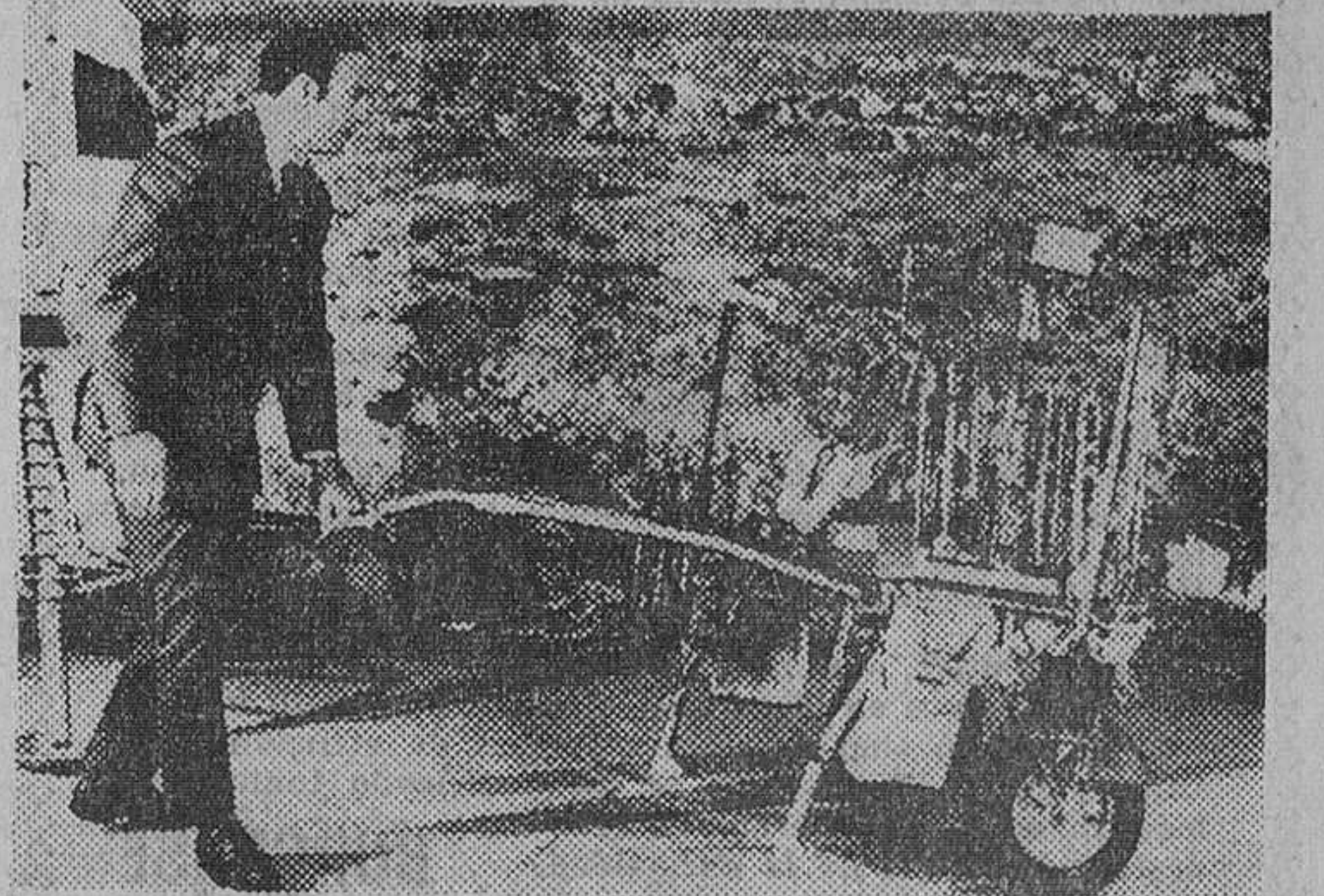
El astronauta norteamericano Edgar D. Mitchell, del «Apolo-14», es fotografiado con la carretilla de veinte libras de peso que utilizarán para la exploración lunar. El curioso vehículo puede transportar 70 libras de equipo, incluyendo seis tubos de perforación, una herramienta para abrir zanjas, dos recogedores geológicos, cuatro bolsas para rocas, un magnetómetro portátil para medir el campo magnético de la Luna y cinco cámaras. Los astronautas Mitchell y Shepard se turnarán para empujar la carretilla durante su segundo paseo por la Luna desde el módulo lunar al cráter del Cono. El lanzamiento del «Apolo-14» está previsto para el día 31 de Enero de 1971. — (Foto FIEL)
